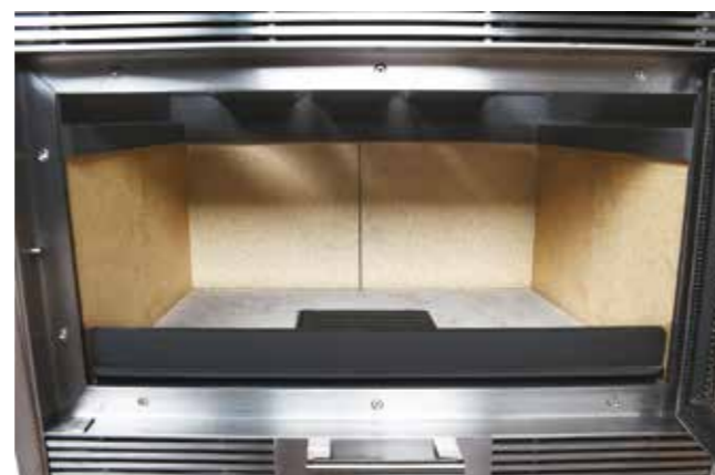
wärmeabstrahlende Feuerraumauskleidung aus Vermiculite
